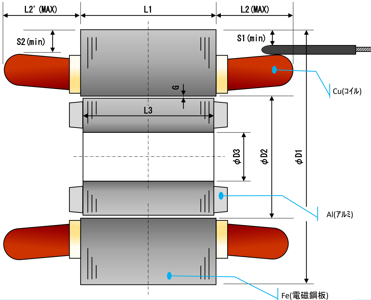
【モータ形状断面図】
