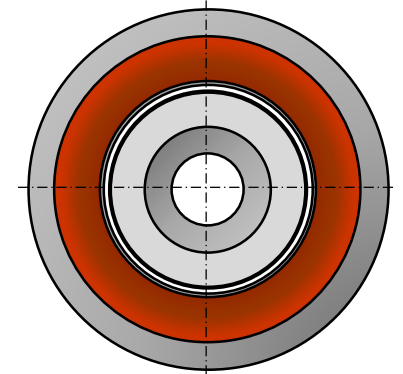
丸コア形状
